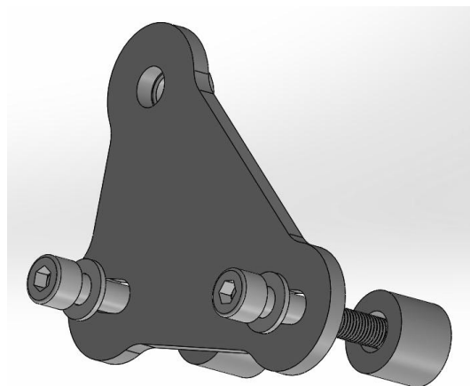
Рис 2 Установленная клетка вид слева
