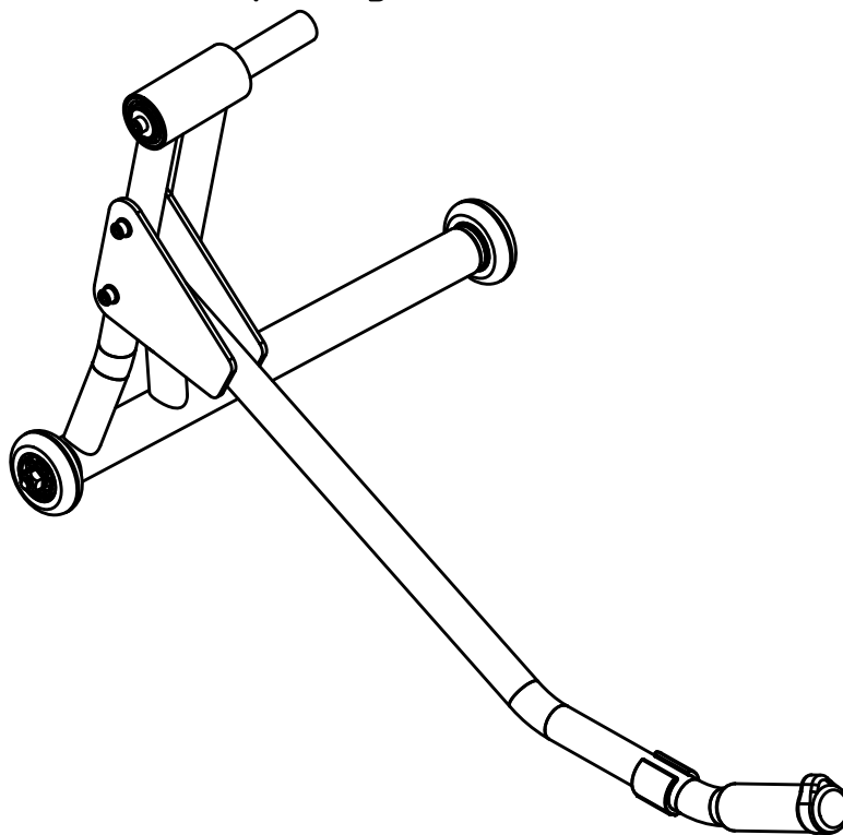
Рис 1 Общий вид собранного консольного мотоподката
