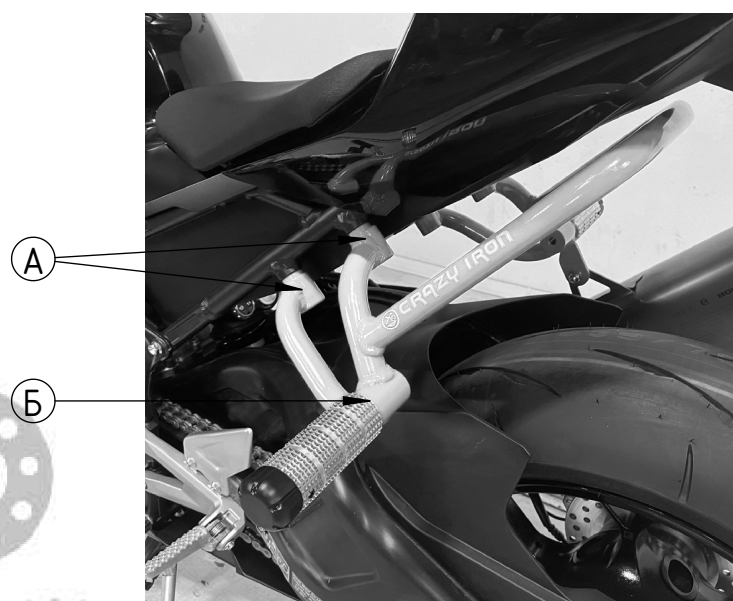
Рис 2 Установленный садкейдж, вид слева.
