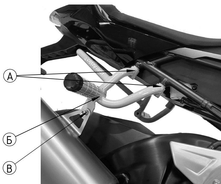
Рис 1 Установленный садкейдж, вид справа
