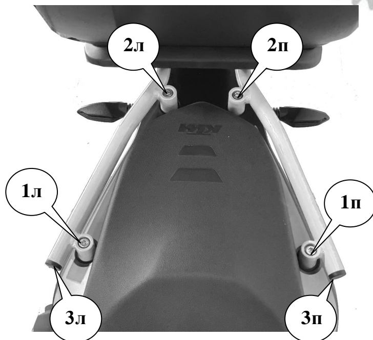
Рис 2 Вид сверху на установленное крепление заднего кофра
