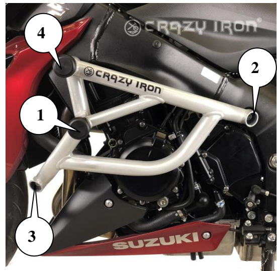
Рис.2. Установленная клетка вид слева
