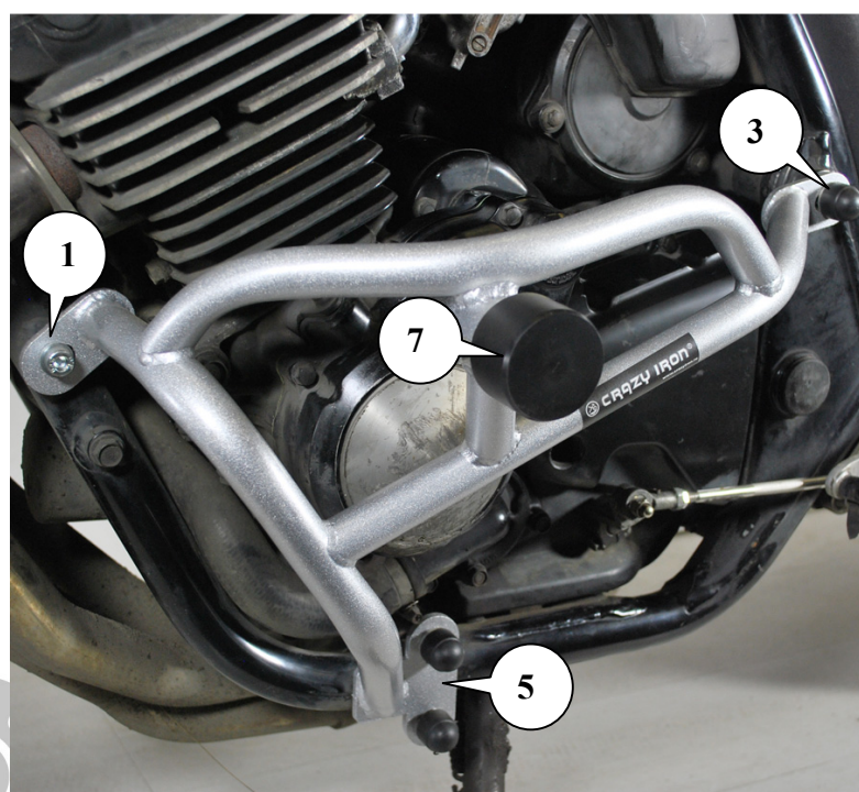
Рис.1. Установленные дуги вид слева
