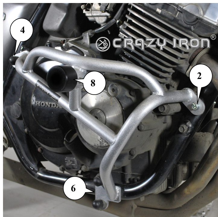
Рис.2. Установленные дуги вид справа
