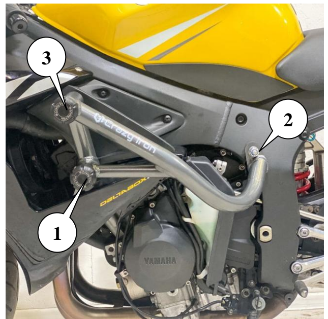
Рис.2. Установленная защита вид слева
