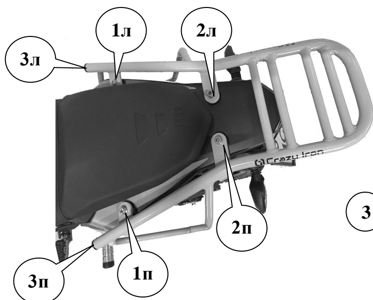
Рис 1 Вид сверху на установленное крепление заднего кофра
