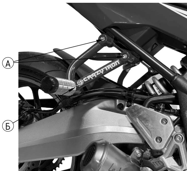
Рис 1 Установленный сабкейдж, вид справа.
