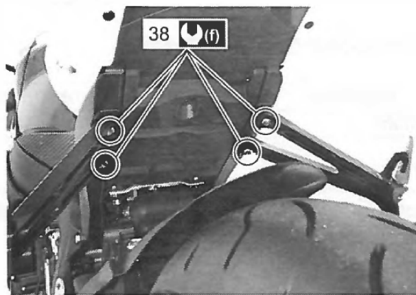
Рис 2 Описание конструкции подножек пассажира из Suzuki GSX-R 600 K6-K7 Service Manual.
