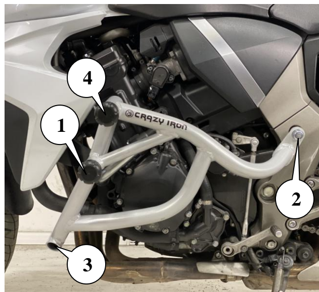
Рис.2. Установленная клетка вид слева
